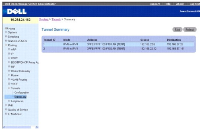
그림 9-44. 터널 요약
