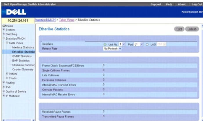
그림 8-2. Etherlike 통계
