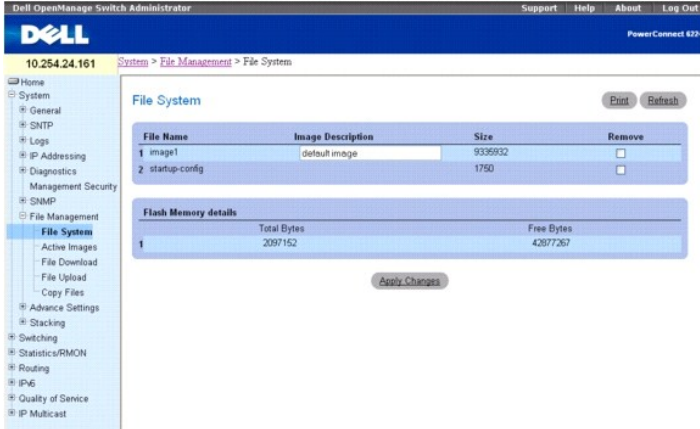
그림 6-72. 파일 시스템
