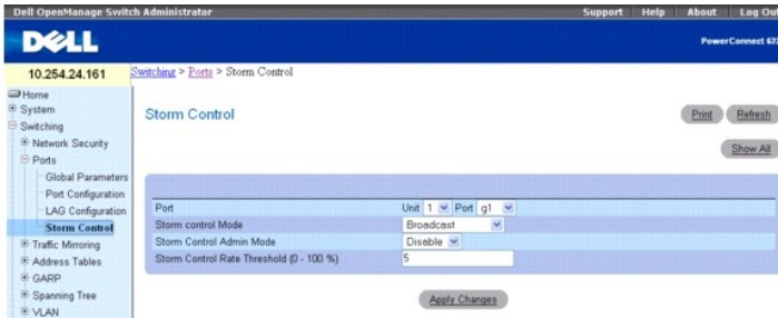
그림 7-24. 뇌우 제어
