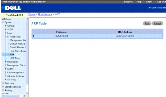
그림 6-25. ARP 표
