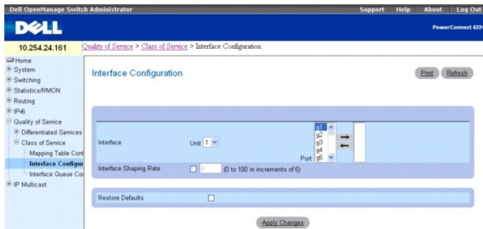
그림 11-19. 인터페이스 구성
